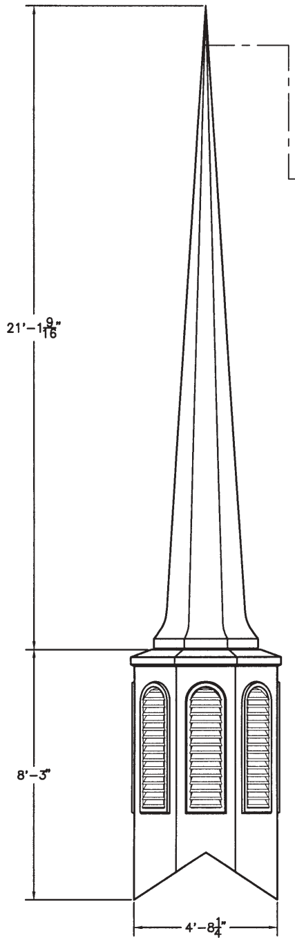
1 ELEVATION E1
