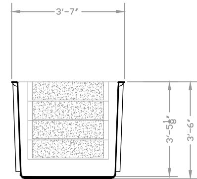
TYP. SECTION
